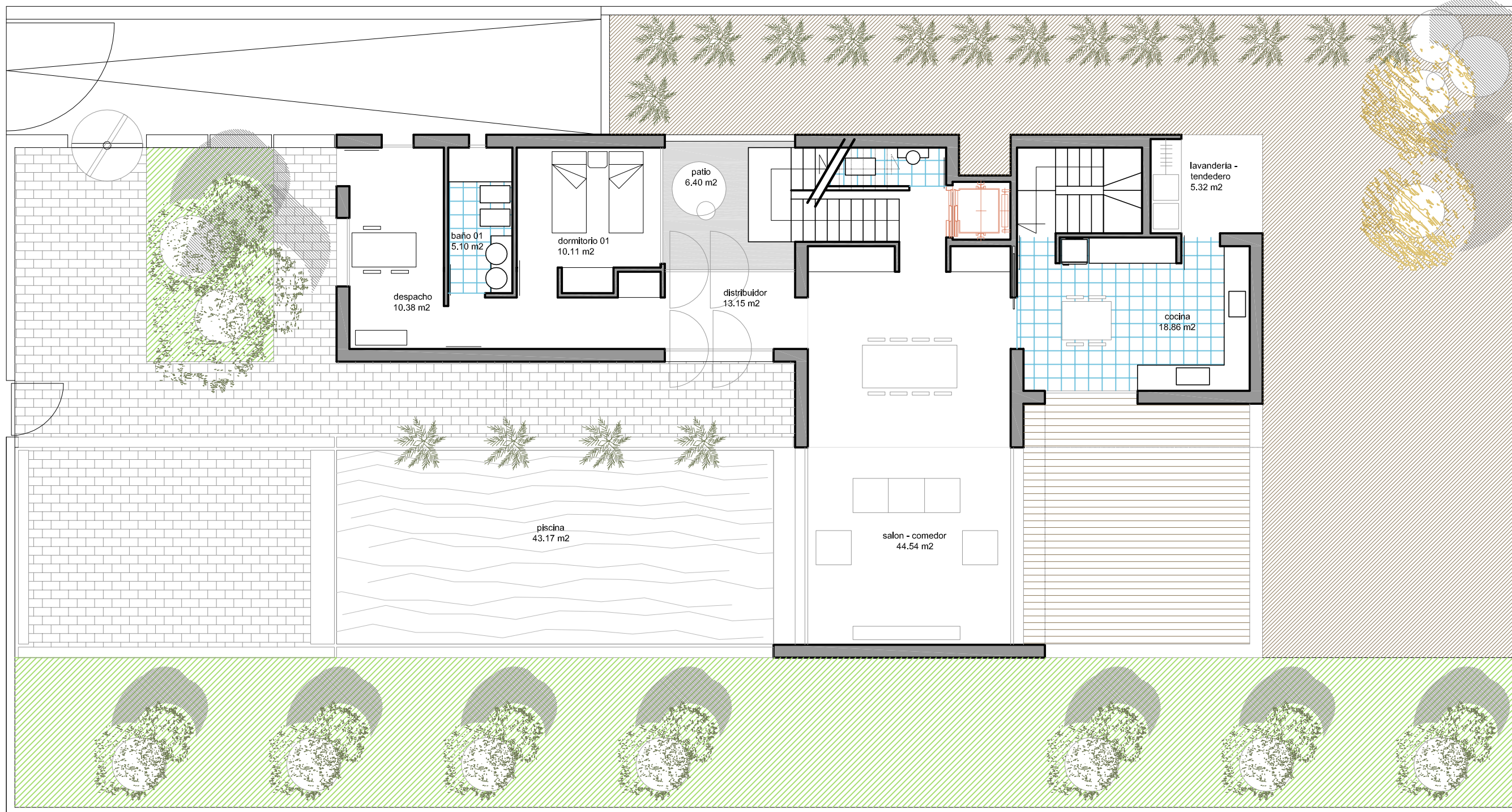
planta baja cota +0.20
