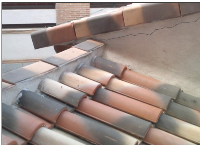
Fig. 4: Fisura característica en la parte superior del borde lateral de una cubierta inclinada (bajo pieza especial de remate).
