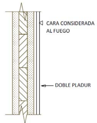
RESISTENCIA AL FUEGO: CLT + DOBLE PLADUR
