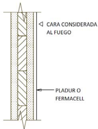
RESISTENCIA AL FUEGO: CLT + PLADUR o CLT + FERMACEL
